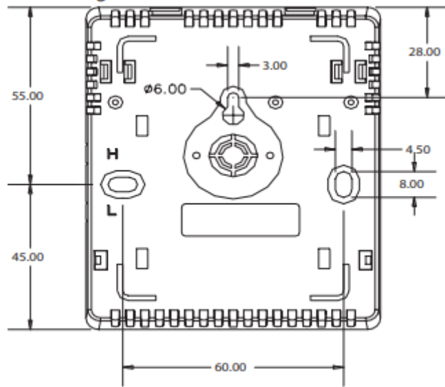
Fig. 1 Dimensions
